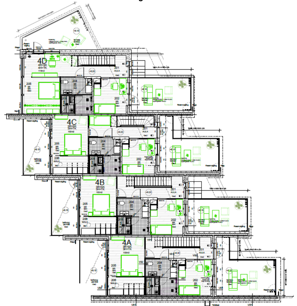
Våning 2
