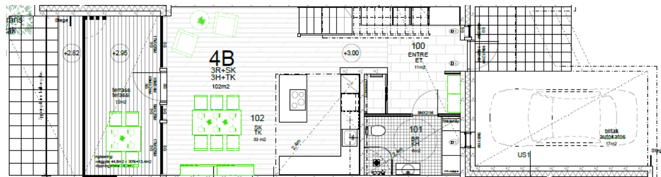
Våning 1
