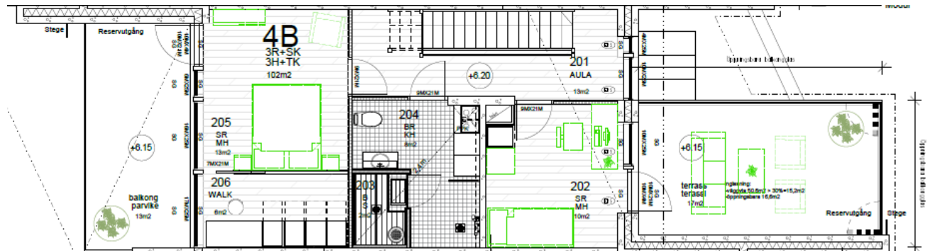
Våning 2
