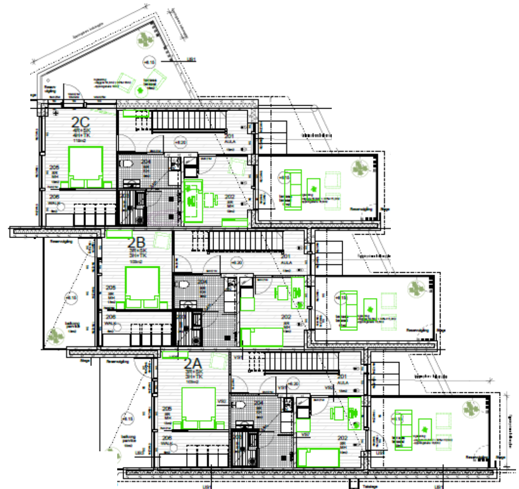
Våning 2
