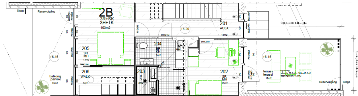
Våning 2
