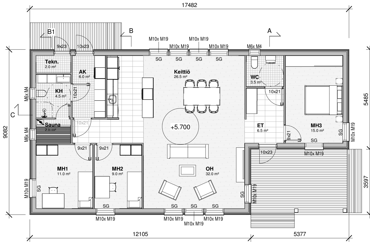
Omakotitalo Pohja 1 : 100
