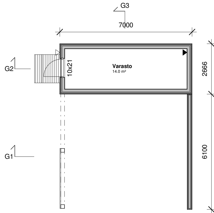
Autokatos Pohja 1 : 100
