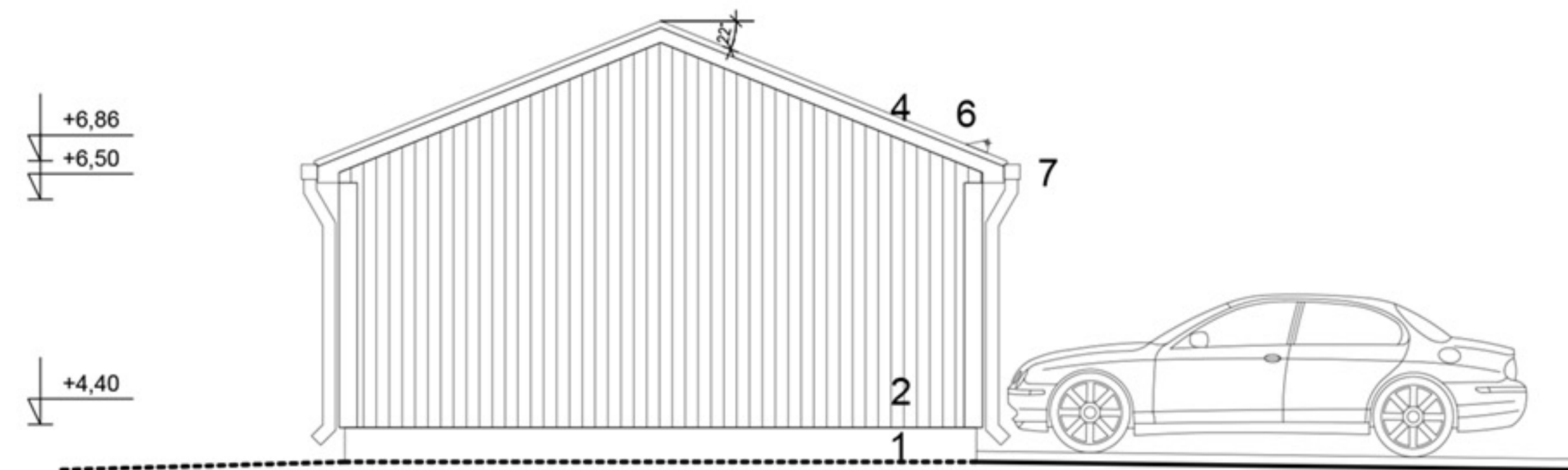
JULKISIVU POHJOISEEN
