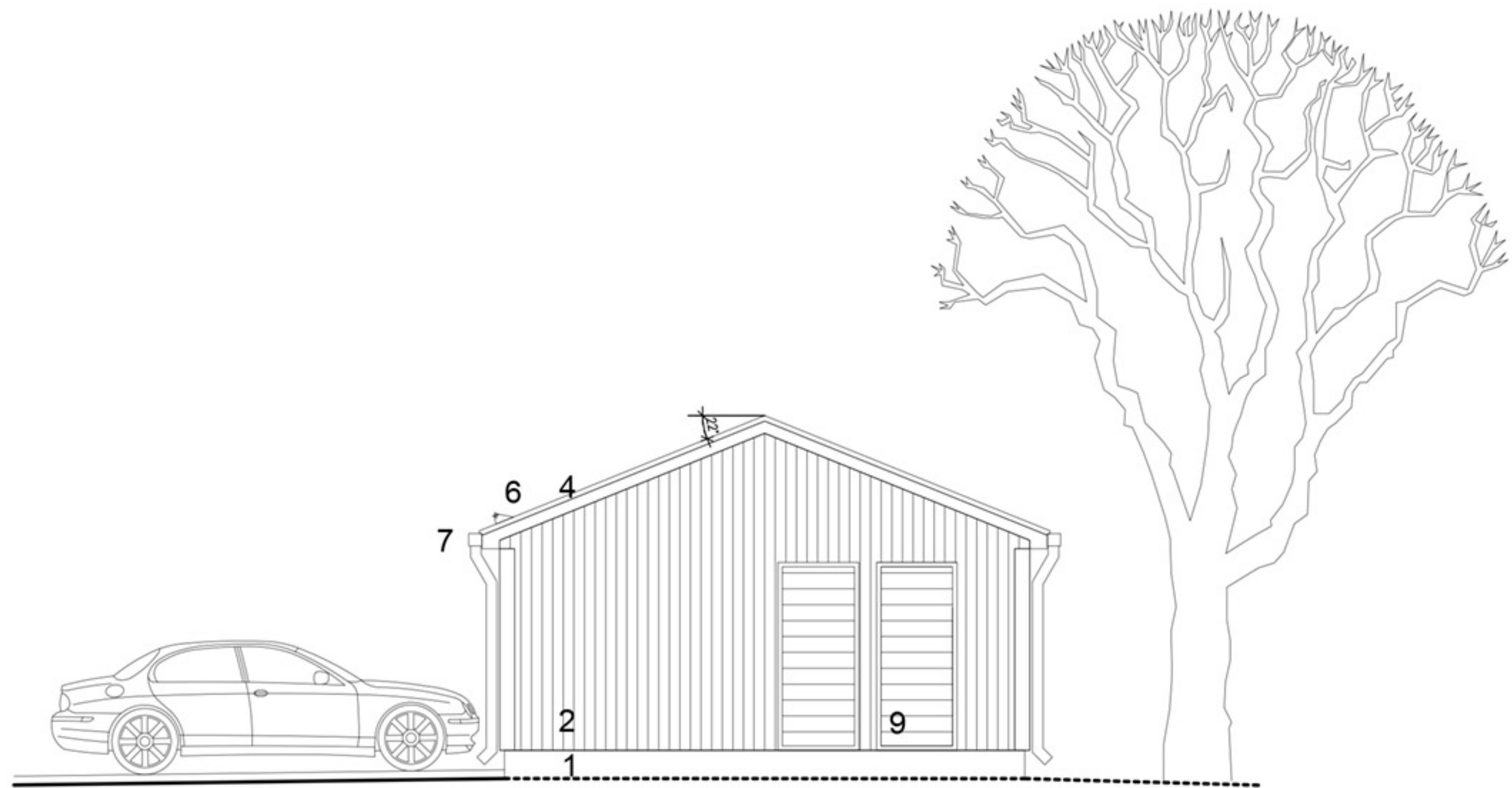
JULKISIVU ETELÄÄN
