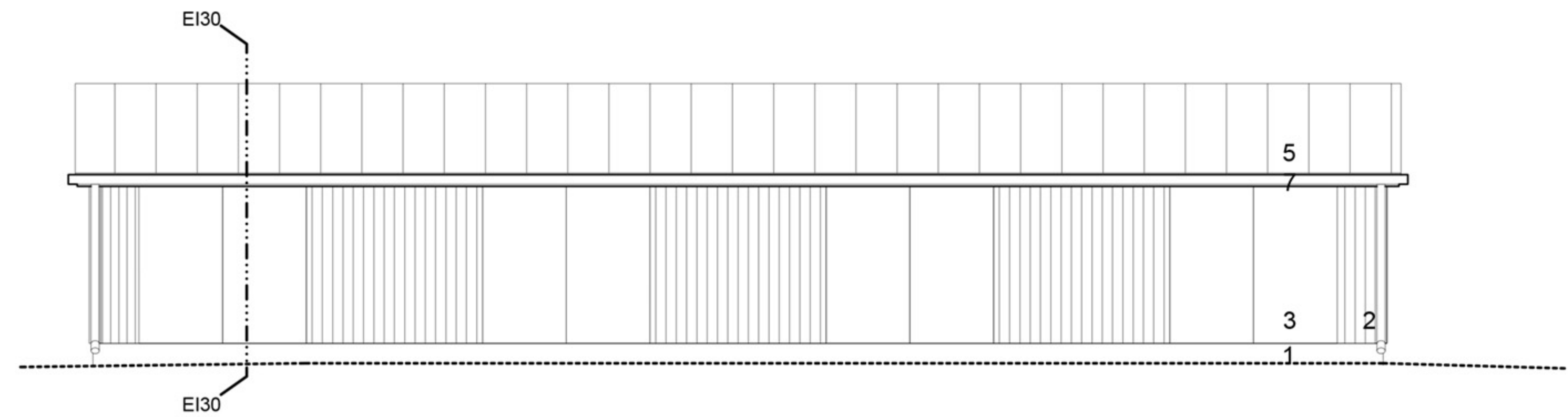
JULKISIVU ITÄÄN
