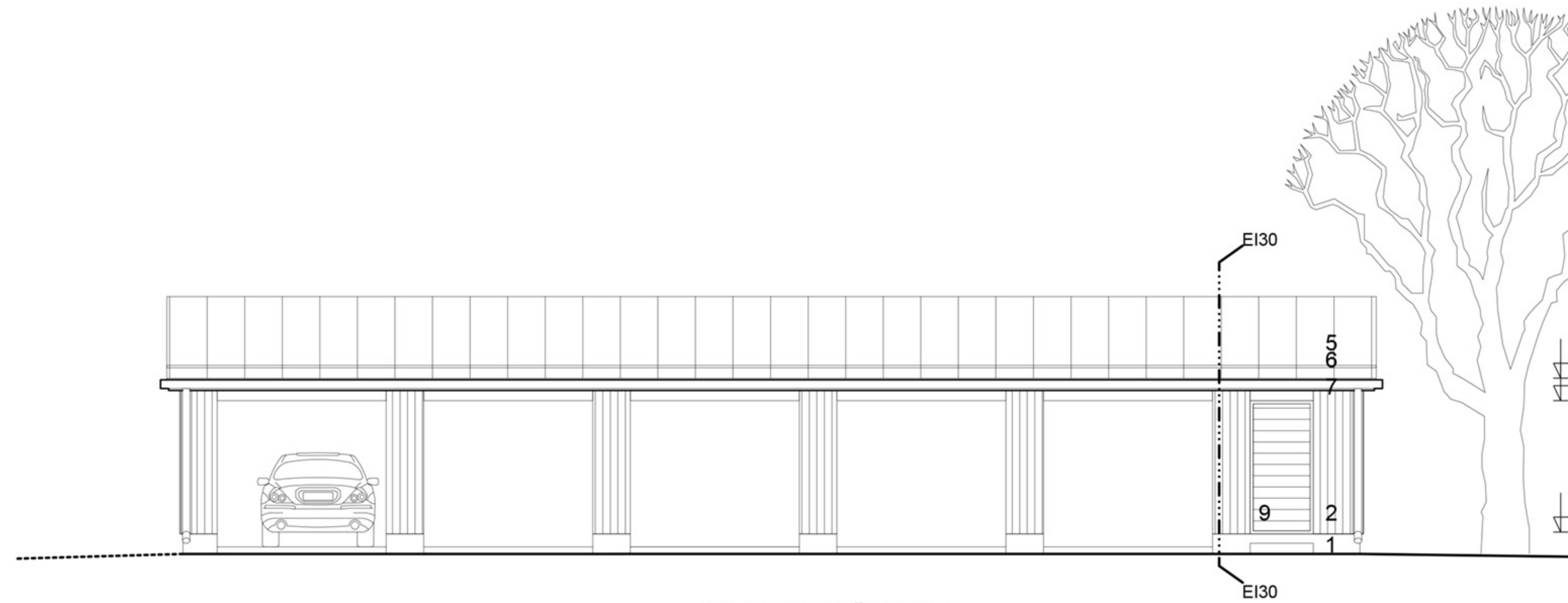
JULKISIVU LÄNTEEN
